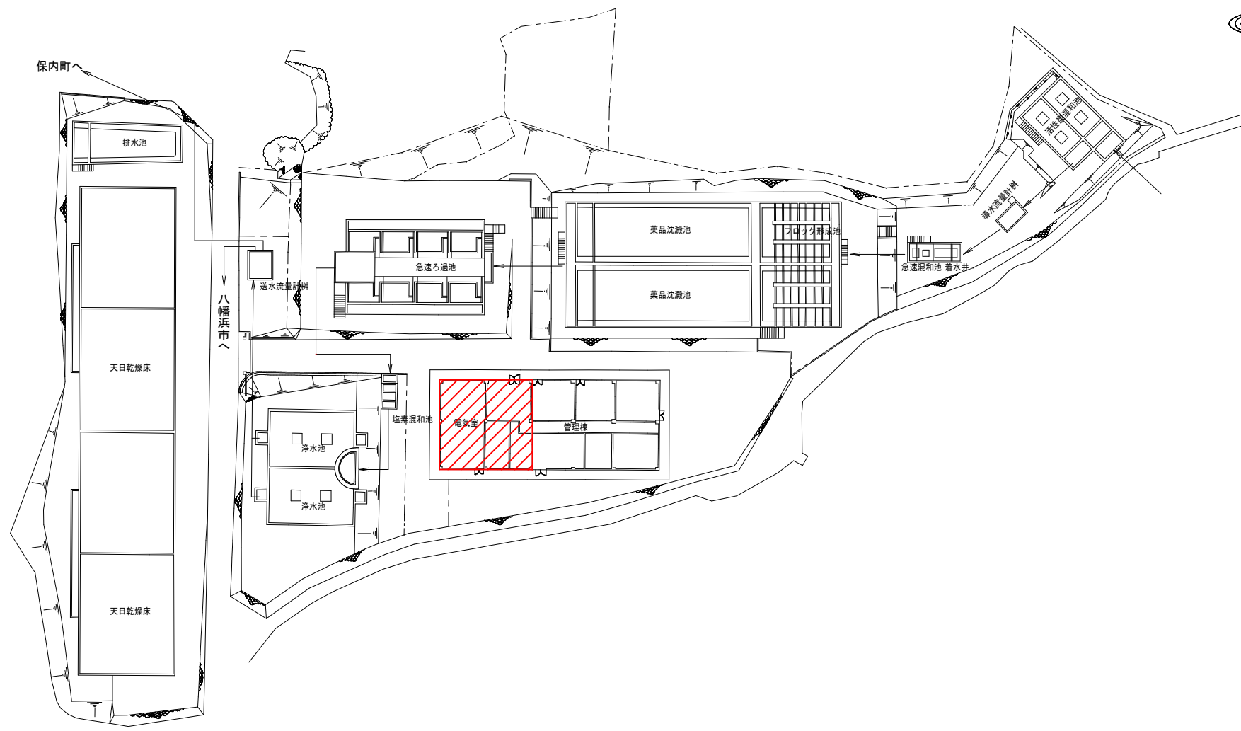
八幡浜浄水場一般平面図 S=1/300
