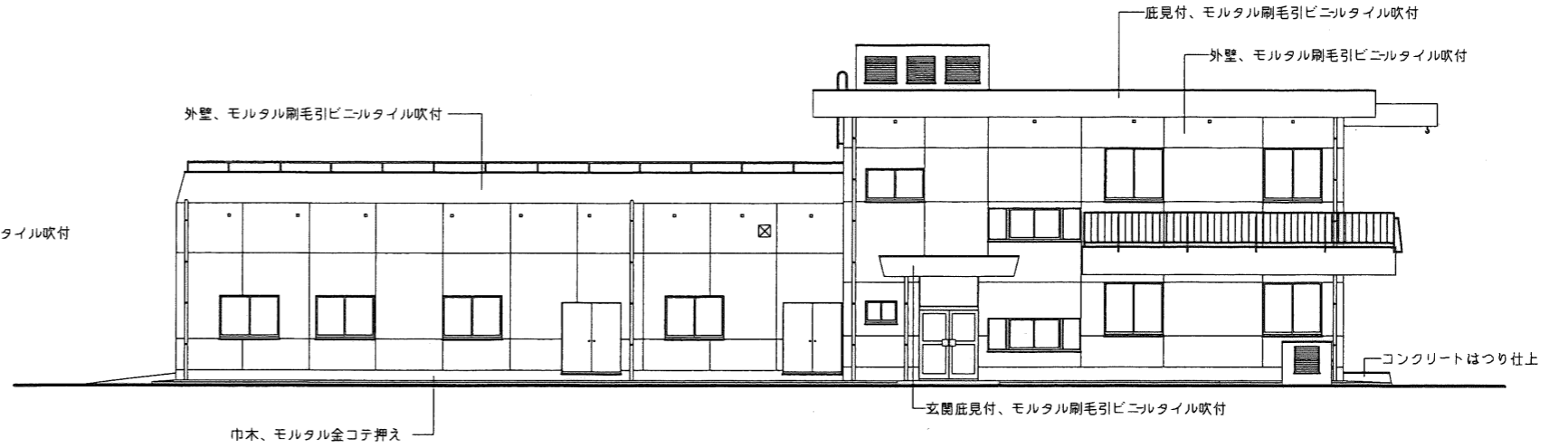
北側立面図 1/100
