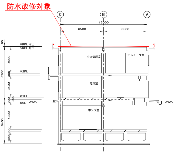
管理本館A-A断面図 S=1/100
