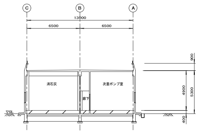
管理本館C-C断面図 S=1/100
