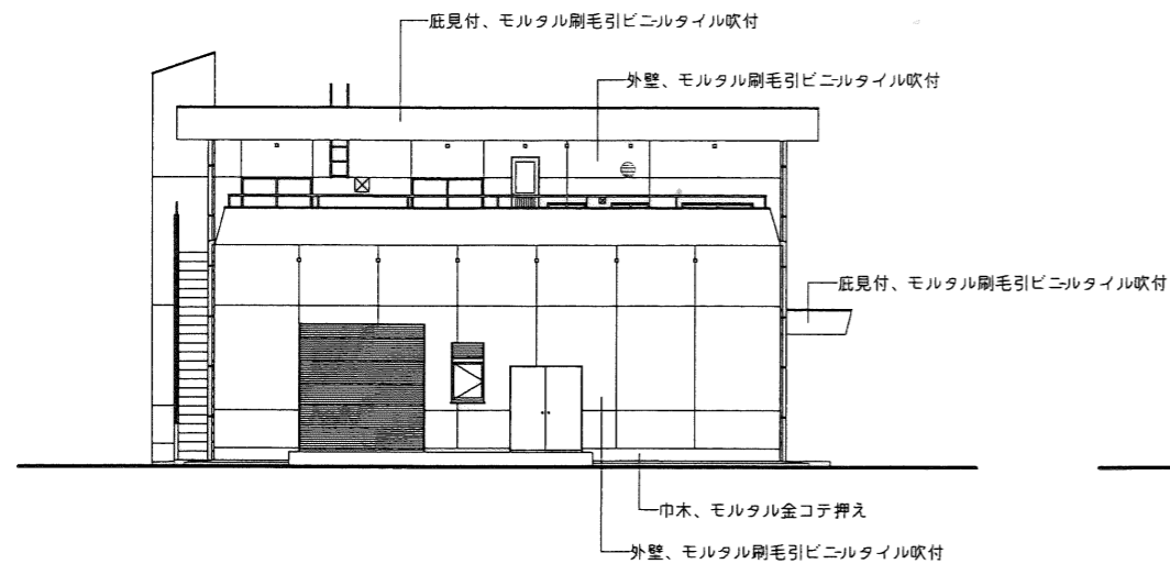
東側立面図 1/100
