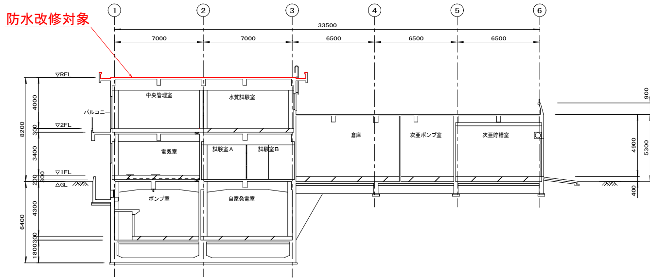
管理本館A-A断面図 S=1/100
