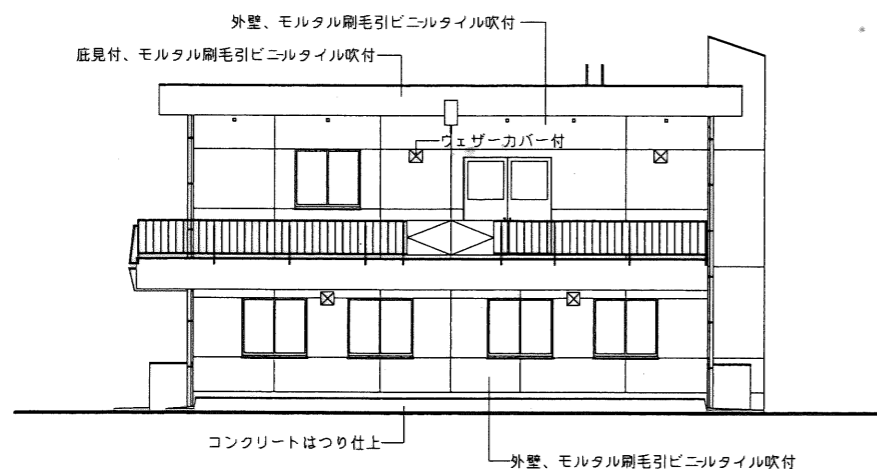
西側立面図 1/100
