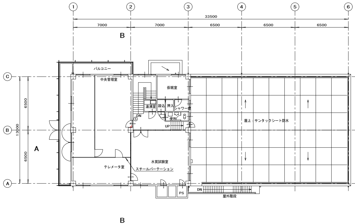
管理本館2階平面図 S=1/100
