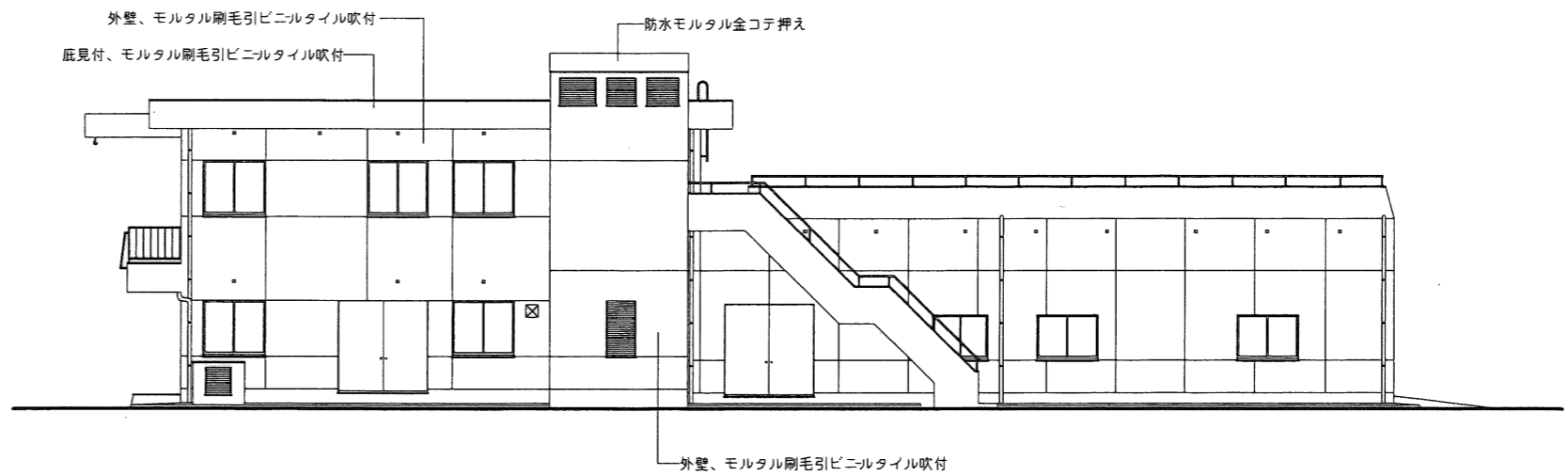
南側立面図 1/100
