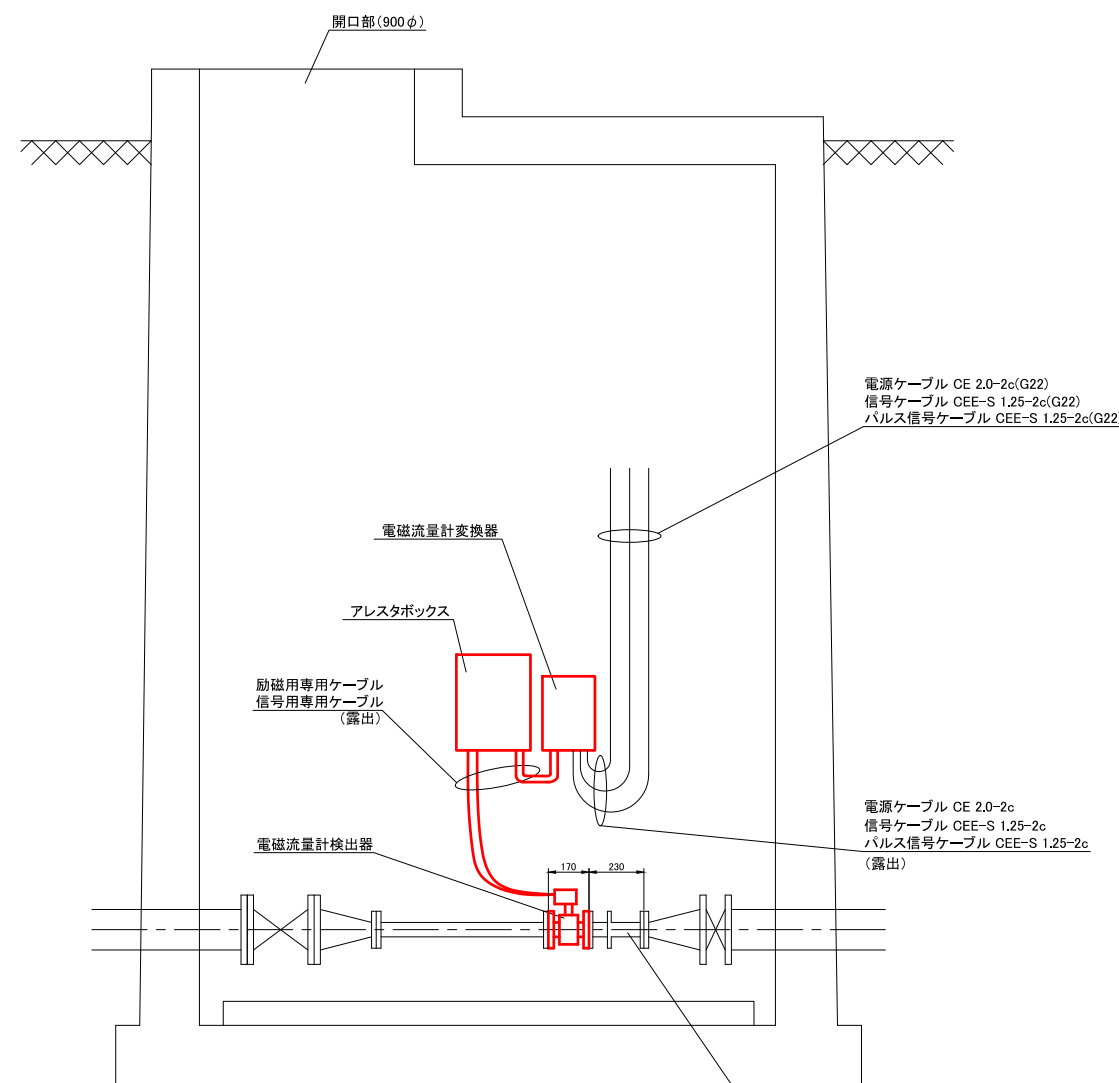
A断面
