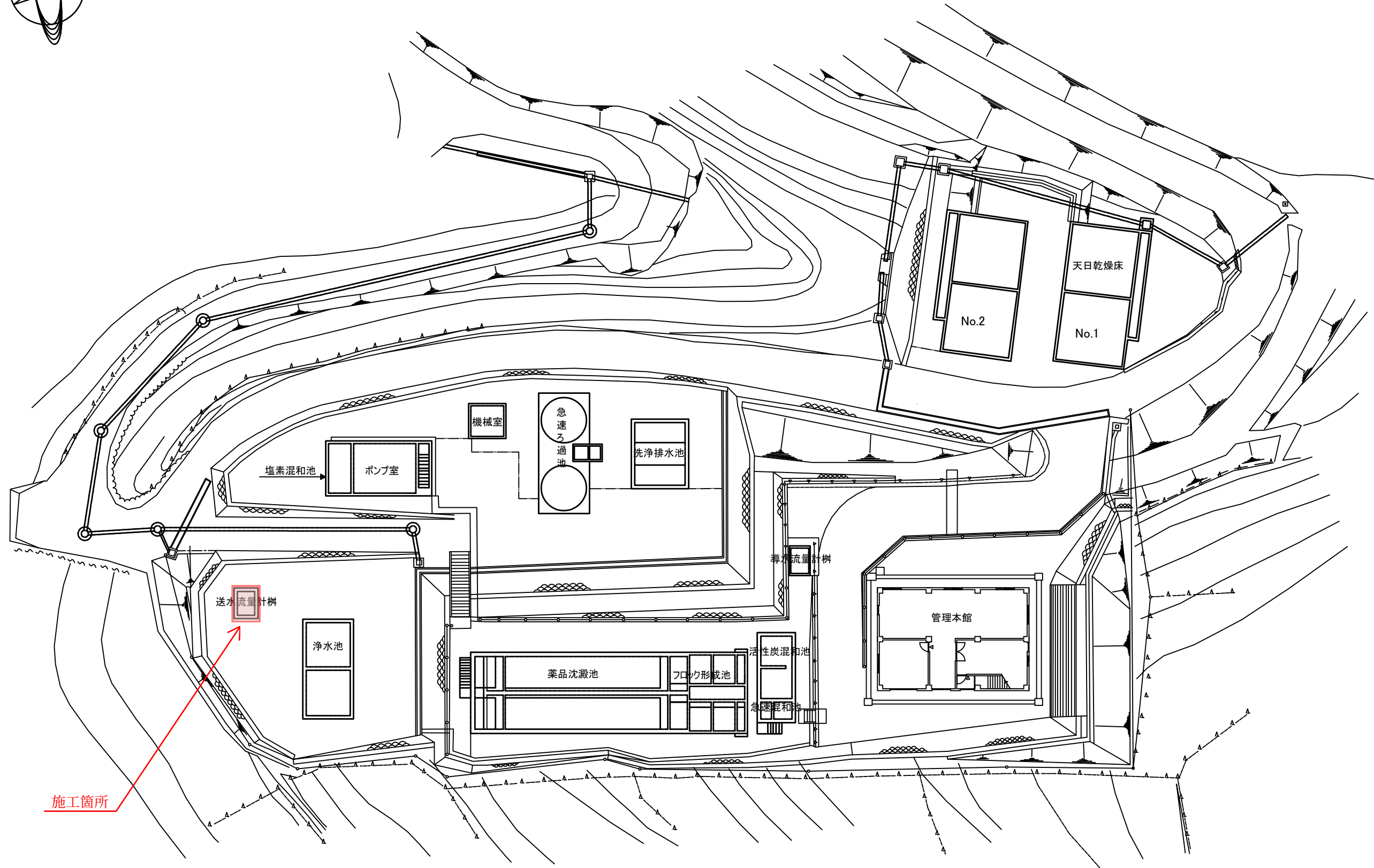
伊方浄水場一般平面図
