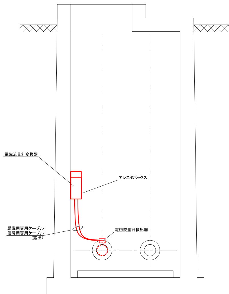
B断面
